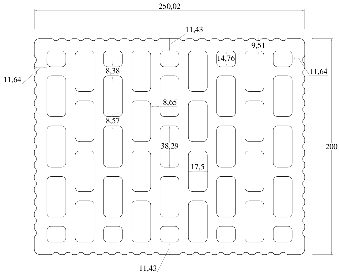
Σχήμα 1. Γεωμετρία οπτόπλινθου
