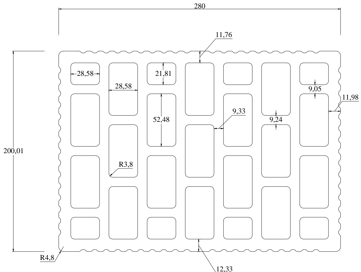
Σχήμα 1. Γεωμετρία οπτόπλινθου
