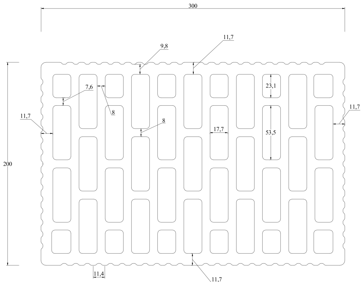
Σχήμα 1. Γεωμετρία οπτόπλινθου
