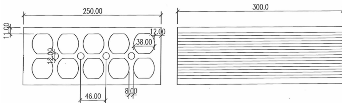
Σχήμα 1. Γεωμετρία οπτόπλινθου
