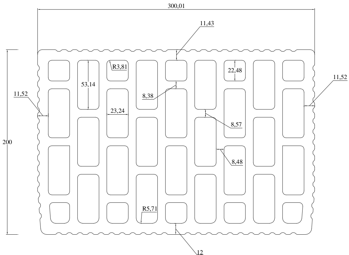
Σχήμα 1. Γεωμετρία οπτόπλινθου
