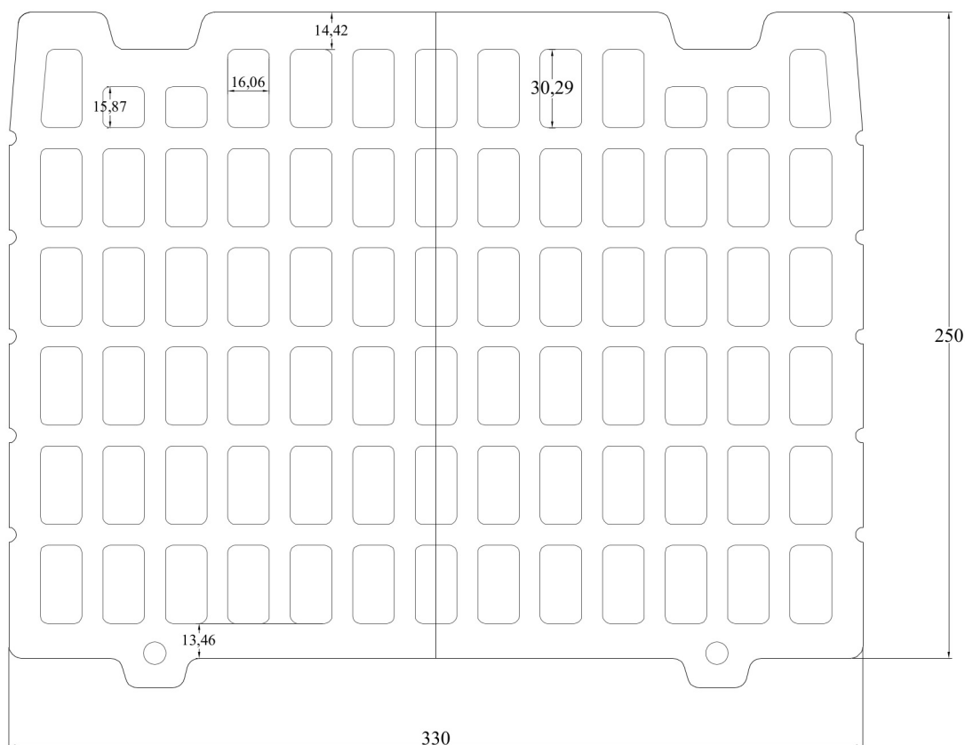
Σχήμα 1. Γεωμετρία οπτόπλινθου
